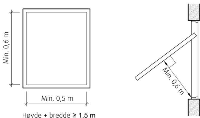
Fig. 8. Minimumsmål på fri åpning til vindu som rømningsvei. Vindu med midtpost må tilfredsstill minimumsmålene på hver side av midtposten.
